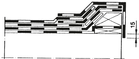
Kuva 3. Saneeraustyö, korotettu räystäs, 3-kermikate.
