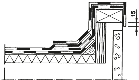
Kuva 5. Räystäs, 2-kermikate.
