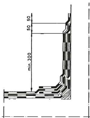
Kuva 9. Seinällenosto, 3-kermikate.
