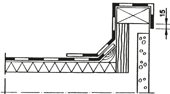
Kuva 4. Räystäs, 1-kermikate.
