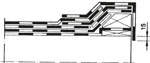
Kuva 3. Saneeraustyö, korotettu räystäs, 3-kermikate.
