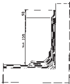
Kuva 8. Seinällenosto, 2-kermikate.
