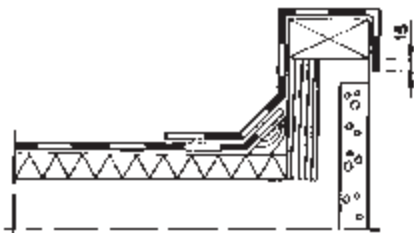
Kuva 4. Räystäs, 1-kermikate.
