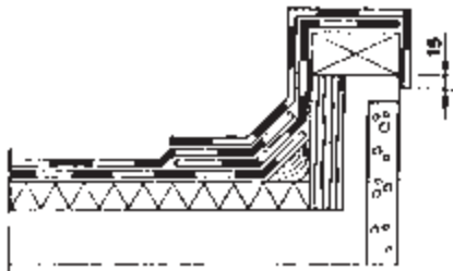
Kuva 5. Räystäs, 2-kermikate.
