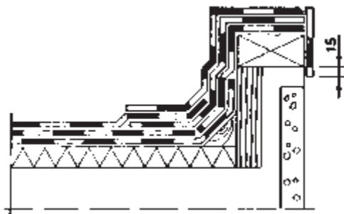
Kuva 6. Rästäs, 3-kermikate.
