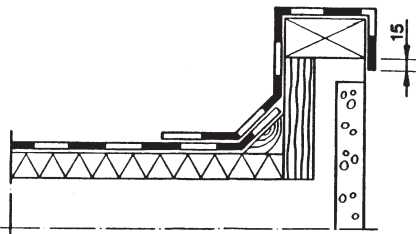
Kuva 4. Räystäs, 1-kermikate.
