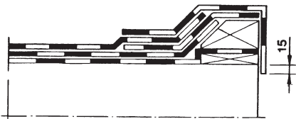
Kuva 2. Saneeraustyö, korotettu räystäs, 2-kermikate.
