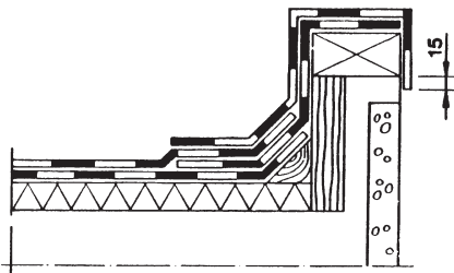
Kuva 5. Räystäs, 2-kermikate.
