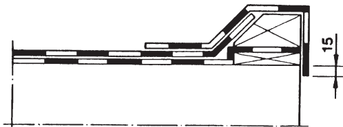
Kuva 1. Saneeraustyö, korotettu räystäs, 1-kermikate.
