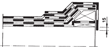
Kuva 3. Saneeraustyö, korotettu räystäs, 3-kermikate.
