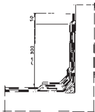
Kuva 8. Seinällenosto, 2-kermikate.
