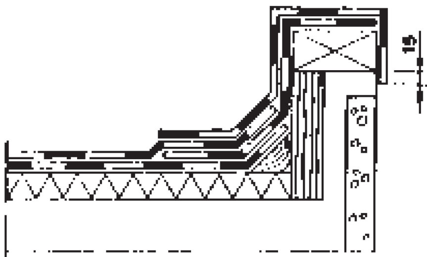
Bild 5. Takskägg, dubbelt tätskikt.
