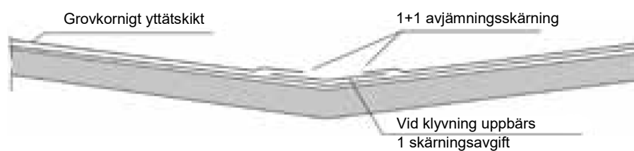
Bild 11. Skärningsavgiften separat för skärningsarbetena i punkterna a och b.
