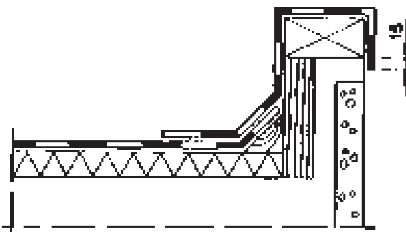
Bild 4. Takskägg, enkelt tätskikt.
