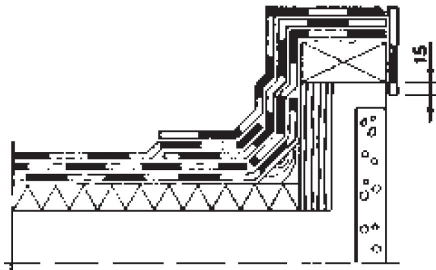
Bild 6. Talskägg, tredubbelt tätskikt.
