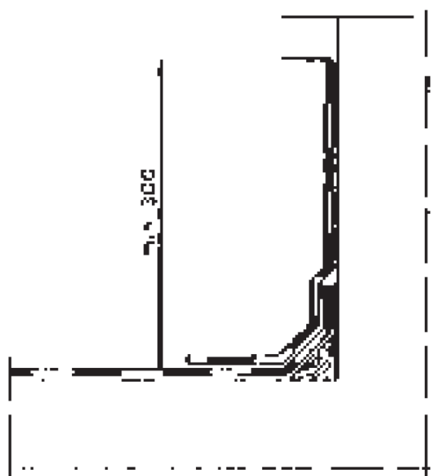
Bild 7. Upp mot vägg, enkelt tätskikt.
