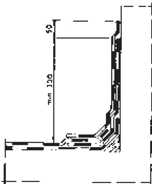
Bild 8. Upp mot vägg, dubbelt tätskikt.
